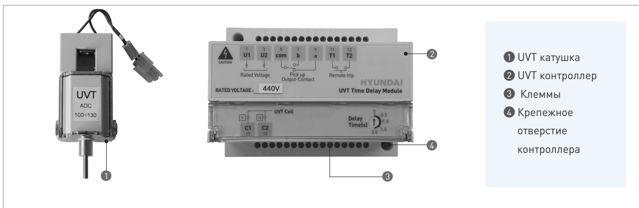
Рис.11 Катушка и контроллер защитного реле минимального напряжения (применимо только для типа с выдержкой по времени)
